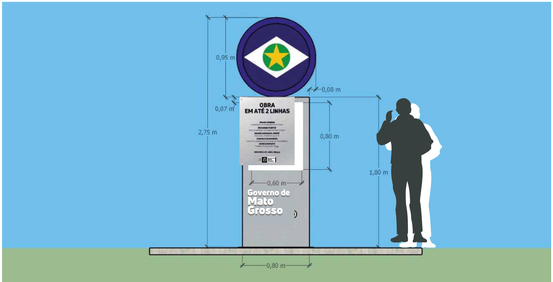
VISTA 01 - TOTEM
