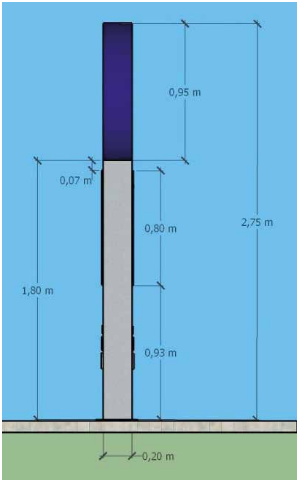
CORTE- TOTEM
